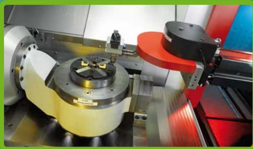
5-Achsen-Fräsmaschine für Graphitelektroden
